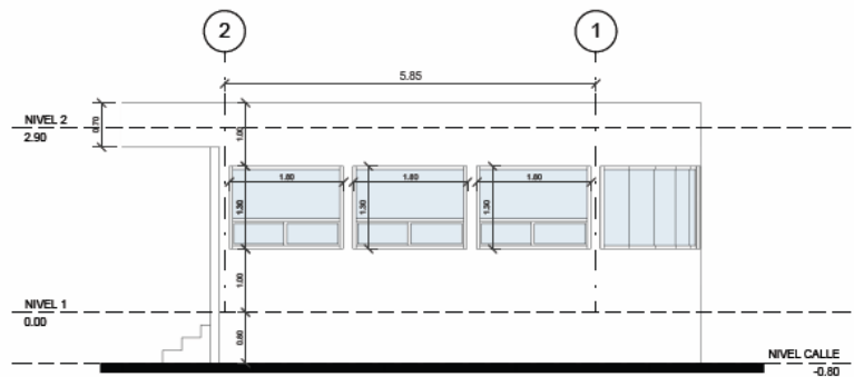
FACHADA LATERAL DERECHA 1 : 50
