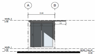
FACHADA A-B 1 : 50
