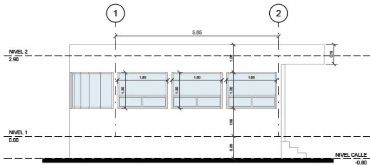
FACHADA LATERAL IZQUIERDA 1 : 50
