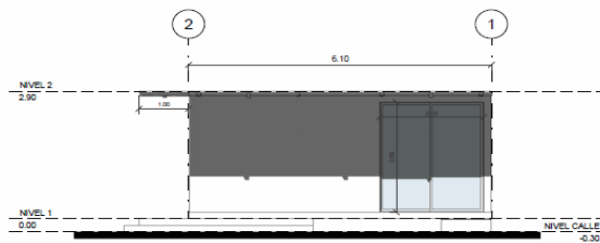
FACHADA 1-2 1 : 50
