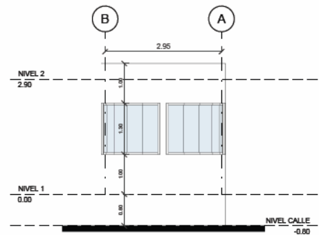
FACHADA TRASERA 1 : 50
