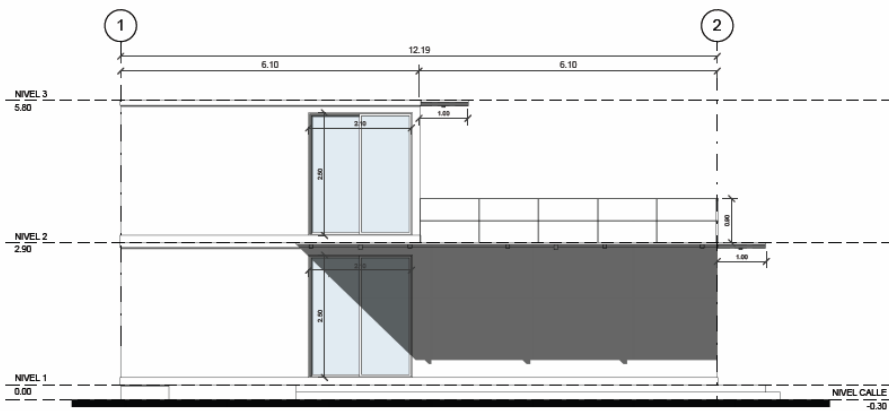
FACHADA 1-2 1 : 50
