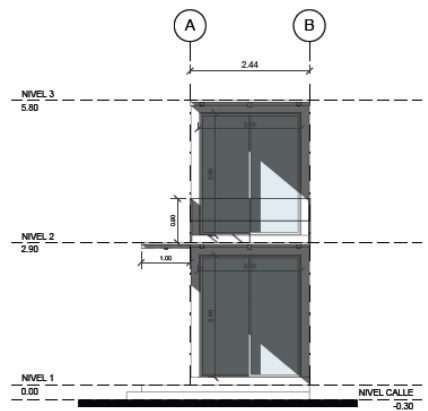
FACHADA A-B 1 : 50
