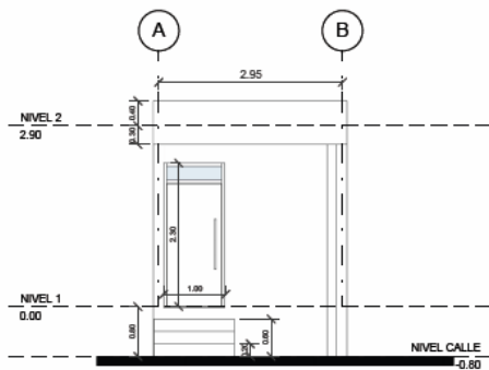
FACHADA FRONTAL 1 : 50
