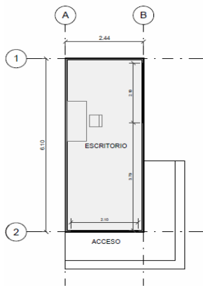
NIVEL 1 1 : 50
